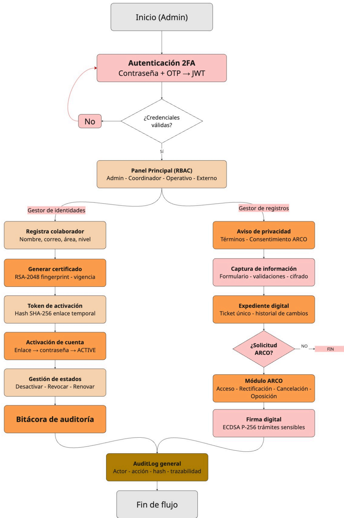
Figure 2: Diagrama de flujo del Gestor de Identidades y Gestor de Registros.
